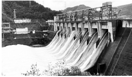
7月8日,浙江新安江水库9个泄洪闸孔全开泄洪,系该水库1959年9月建成以来的首次
